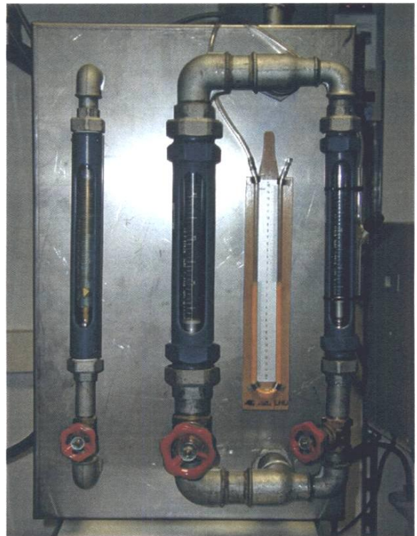
Bild 5b: Prüfstand-Steuerung (Wasser- u. Luftmenge)
