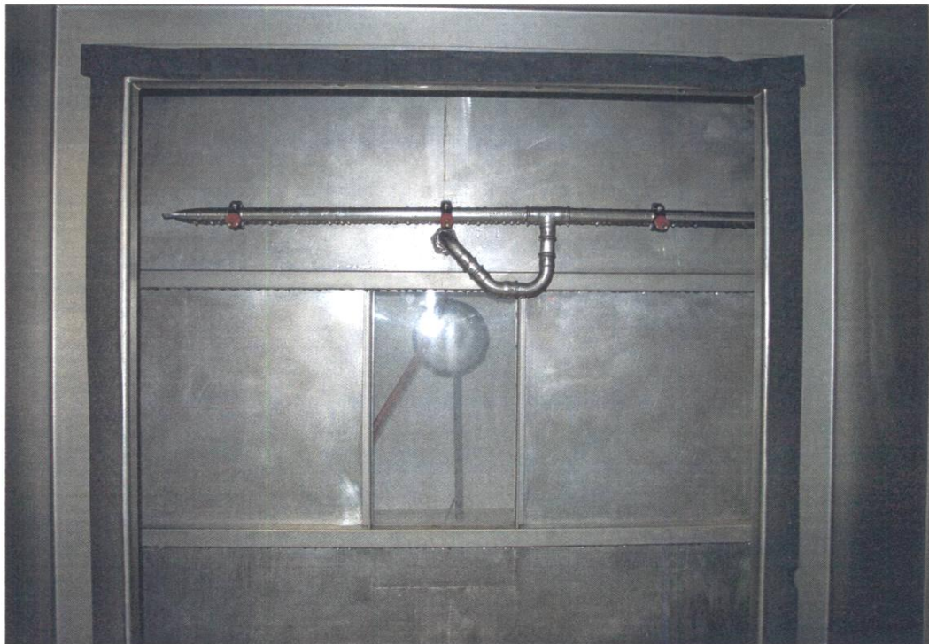
Bild 4: Offener Prüfstand mit Anordnung der drei wassersprühenden Düsen
