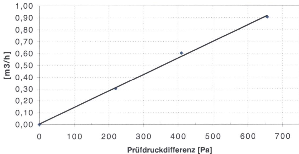
Bild 1: Grafische Darstellung der Prüfstandundichtigkeit (Längsfugen)
