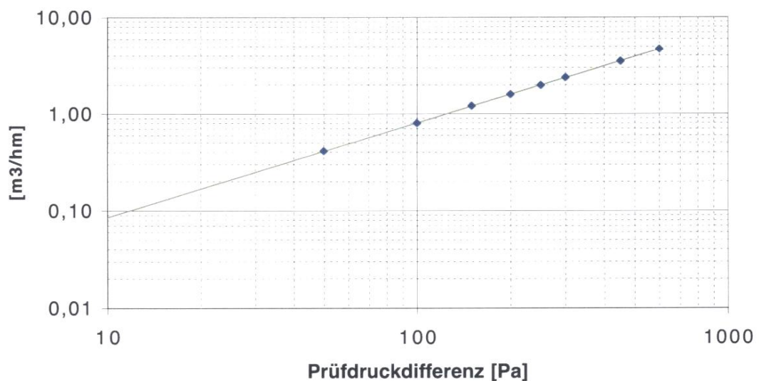
Bild 2: Grafische Darstellung der längenbezogenen Luftdurchlässigkeit (Längsfugen)
